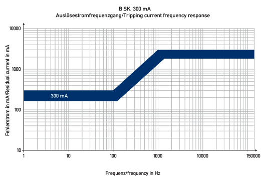
Diagramme Fehlerstromschutzschalter DFS 4 080-4/0,30-B SK NA
