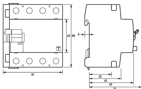
Mazeichnung Fehlerstromschutzschalter DFS 4 080-4/0,30-B SK NA
