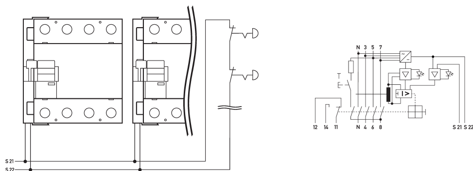
Schaltungsbeispiel Fehlerstromschutzschalter DFS 4 080-4/0,30-B SK NA
