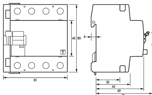
Maßzeichnung Fehlerstromschutzschalter DFS 4 080-4/0,03-B SK NA
