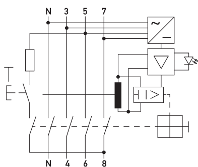
Schaltungsbeispiel Fehlerstromschutzschalter DFS 4 063-4/0,50-B SK ISO HD
