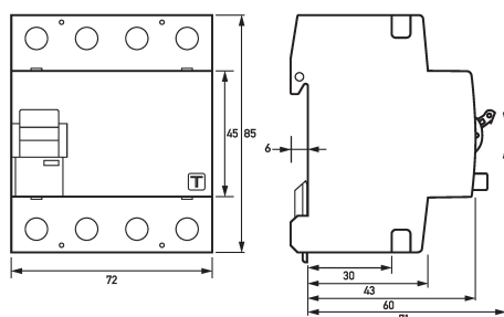
Maßzeichnung Fehlerstromschutzschalter DFS 4 063-4/0,30-B SK ISO HD
