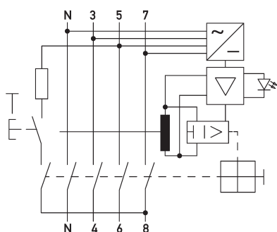
Schaltungsbeispiel Fehlerstromschutzschalter DFS 4 063-4/0,10-B NK HD
