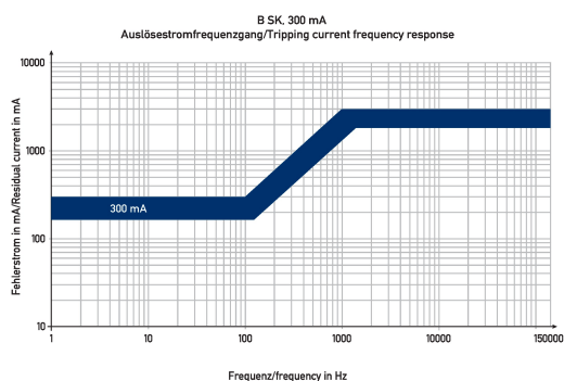
Diagramme Fehlerstromschutzschalter DFS 4 040-4/0,30-B SK MI HD
