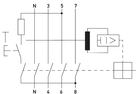
Schaltungsbeispiel Fehlerstromschutzschalter DFS 4 040-4/0,03-A HT HD75
