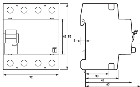
Maßzeichnung Fehlerstromschutzschalter DFS 4 040-4/0,03-A HT HD75
