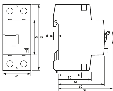
Maßzeichnung Fehlerstromschutzschalter DFS 2 025-2/0,10-PV HD
