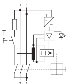
Schaltungsbeispiel Fehlerstromschutzschalter DFS 2 025-2/0,10-PV
