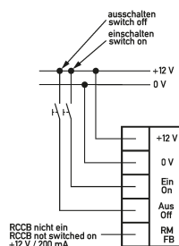
Schaltungsbeispiel automatisch wiedereinschaltende Einrichtungen DFA 3 012DC-3
