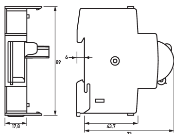
Maßzeichnung automatisch wiedereinschaltende Einrichtungen DFA 3 012DC-3
