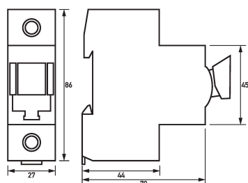
Mazeichnung Sicherungslasttrennschalter Tytan II Do-63-1/E
