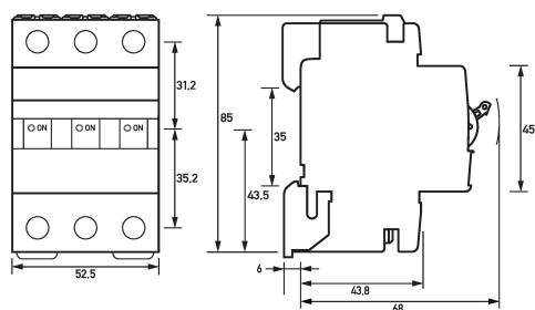
Maßzeichnung Leitungsschutzschalter DLS 6hsl C16-3
