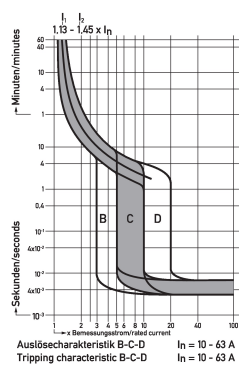
Diagramme Leitungsschutzschalter DLS 6hsl C16-3
