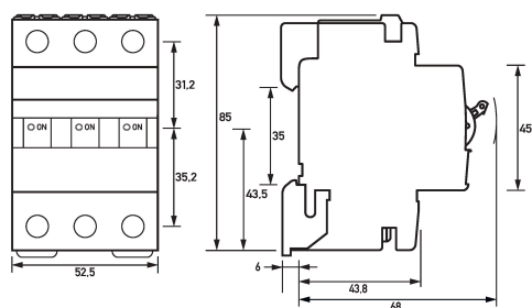
Maßzeichnung Leitungsschutzschalter DLS 6hsl B16-3
