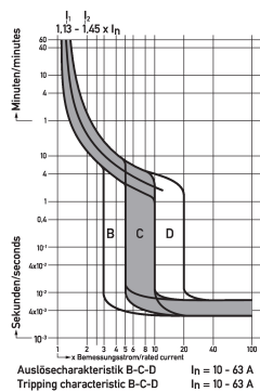
Diagramme Leitungsschutzschalter DLS 6hsl B20-1
