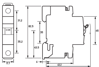
Maßzeichnung Leitungsschutzschalter DLS 6i B16-1 RT
