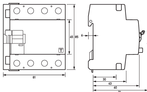
Maßzeichnung Fehlerstromschutzschalter DFS 4 063-4/0,03-A EV NA HD
