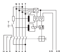
Schaltungsbeispiel Fehlerstromschutzschalter DFS 4 063-4/0,03-A EV NA HD
