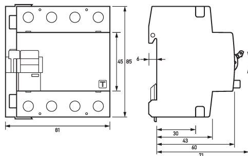
Maßzeichnung Fehlerstromschutzschalter DFS 4 063-4/0,03-A EV NA
