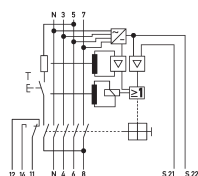
Schaltungsbeispiel Fehlerstromschutzschalter DFS 4 063-4/0,03-A EV NA
