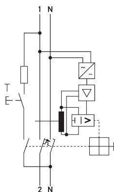
Schaltungsbeispiel FI-/LS-Kombinationen DRCBO 4 C32/0,10/1N-HP
