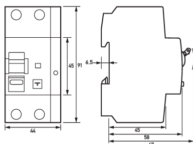
Maßzeichnung FI-/LS-Kombinationen DRCBO 4 C25/0,10/1N-HP
