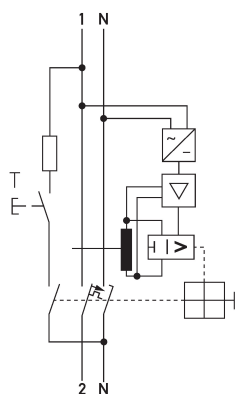
Schaltungsbeispiel FI-/LS-Kombinationen DRCBO 4 C32/0,30/1N-HP
