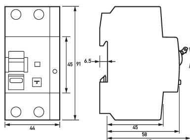
Maßzeichnung FI-/LS-Kombinationen DRCBO 4 C32/0,30/1N-HP
