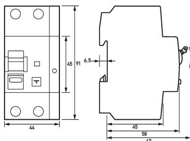
Maßzeichnung FI-/LS-Kombinationen DRCBO 4 C32/0,03/1N-HP
