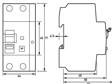
Maßzeichnung FI-/LS-Kombinationen DRCBO 4 C25/0,03/1N-HP
