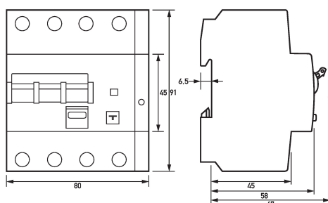
Maßzeichnung FI-/LS-Kombinationen DRCBO 4 C32/0,10/3N-HP
