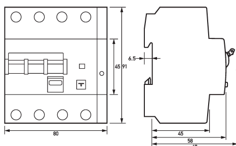
Maßzeichnung FI-/LS-Kombinationen DRCBO 4 C16/0,10/3N-HP
