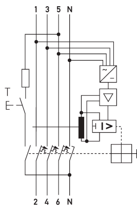
Schaltungsbeispiel FI-/LS-Kombinationen DRCBO 4 C25/0,30/3N-HP
