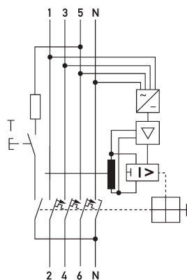
Schaltungsbeispiel FI-/LS-Kombinationen DRCBO 4 C16/0,30/3N-HP
