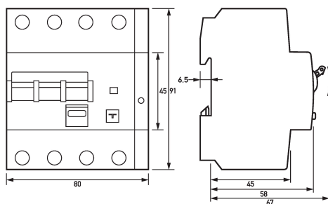
Maßzeichnung FI-/LS-Kombinationen DRCBO 4 C32/0,03/3N-HP
