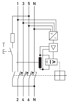
Schaltungsbeispiel FI-/LS-Kombinationen DRCBO 4 C32/0,03/3N-HP
