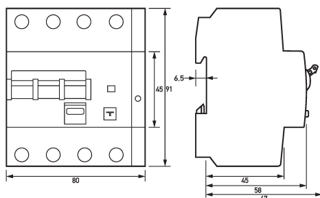
Maßzeichnung FI-/LS-Kombinationen DRCBO 4 C16/0,03/3N-HP
