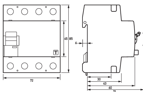
Maßzeichnung Fehlerstromschutzschalter DFS 4 063-4/0,30-HP HD
