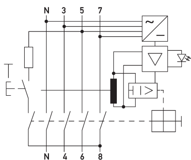
Schaltungsbeispiel Fehlerstromschutzschalter DFS 4 063-4/0,10-HP
