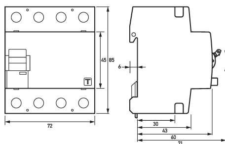
Maßzeichnung Fehlerstromschutzschalter DFS 4 063-4/0,03-HP HD
