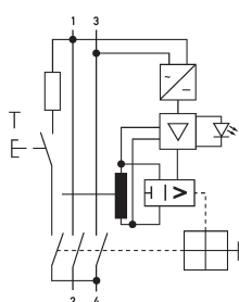
Schaltungsbeispiel Fehlerstromschutzschalter DFS 2 040-2/0,30-HP HD
