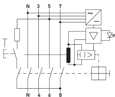
Schaltungsbeispiel Fehlerstromschutzschalter DFS 4 040-4/0,03-HP HD
