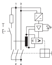
Schaltungsbeispiel Fehlerstromschutzschalter DFS 2 040-2/0,03-HP
