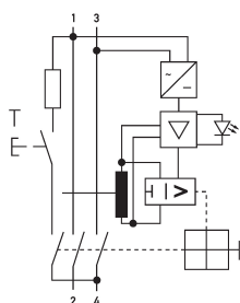
Schaltungsbeispiel Fehlerstromschutzschalter DFS 2 025-2/0,10-HP
