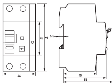
Maßzeichnung FI-/LS-Kombinationen DRCBO 4 C32/0,10/1N-PV
