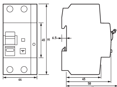
Maßzeichnung FI-/LS-Kombinationen DRCBO 4 C32/0,30/1N-PV
