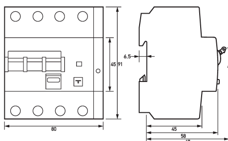
Maßzeichnung FI-/LS-Kombinationen DRCBO 4 C32/0,10/3N-PV
