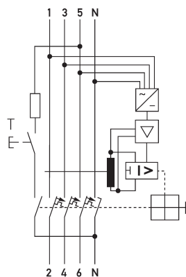
Schaltungsbeispiel FI-/LS-Kombinationen DRCBO 4 C25/0,10/3N-PV
