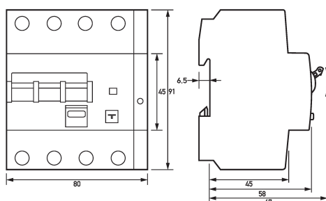
Maßzeichnung FI-/LS-Kombinationen DRCBO 4 C25/0,10/3N-PV
