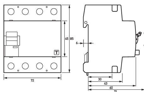
Maßzeichnung Fehlerstromschutzschalter DFS 4 063-4/0,10-PV HD
