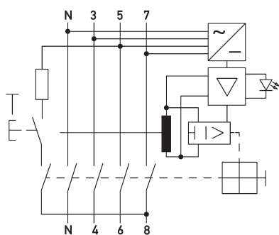
Schaltungsbeispiel Fehlerstromschutzschalter DFS 4 063-4/0,10-PV HD
