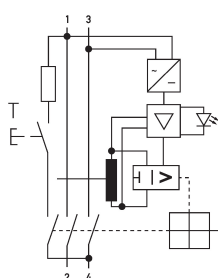
Schaltungsbeispiel Fehlerstromschutzschalter DFS 2 040-2/0,30-PV HD
