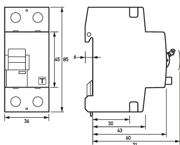
Maßzeichnung Fehlerstromschutzschalter DFS 2 040-2/0,30-PV HD
