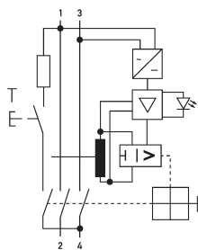
Schaltungsbeispiel Fehlerstromschutzschalter DFS 2 040-2/0,30-PV
