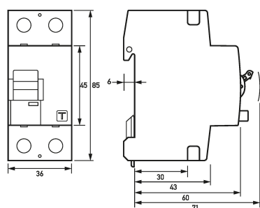
Maßzeichnung Fehlerstromschutzschalter DFS 2 040-2/0,10-PV HD
