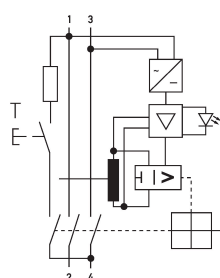
Schaltungsbeispiel Fehlerstromschutzschalter DFS 2 040-2/0,10-PV HD
