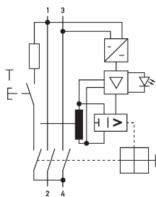
Schaltungsbeispiel Fehlerstromschutzschalter DFS 2 040-2/0,10-PV
