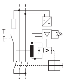
Schaltungsbeispiel Fehlerstromschutzschalter DFS 2 025-2/0,30-PV HD
