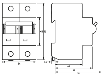
Maßzeichnung Gruppenansicht
