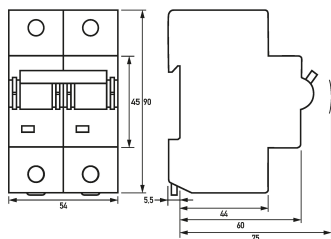
Maßzeichnung Gruppenansicht
