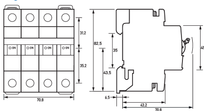
Maßzeichnung Gruppenansicht
