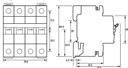
Maßzeichnung Gruppenansicht
