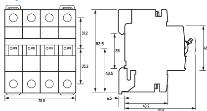
Maßzeichnung Gruppenansicht
